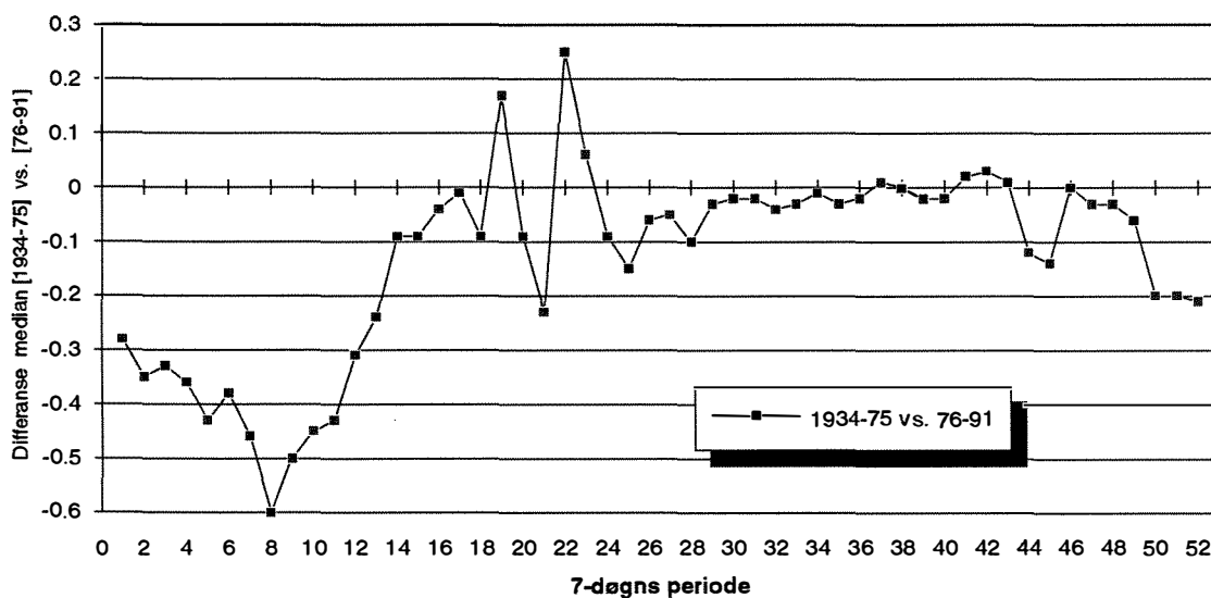
Figur 4. Differanser i median vannstand (beregnet ut ifra ukeverdier) for Øyeren hhv. før utsprenkningene ved Mørkfoss (1934-75) og etter (1976-91)
