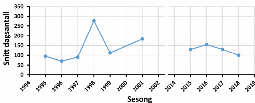
Figur 5: Utviklingen i dagstallet for antall vadere på Årnestangens sørspiss. Kurven er basert på tellinger utført i perioden 15.7-15.9 for årene 1995-2001 og 2015-2018 (n=88; feltdager).
