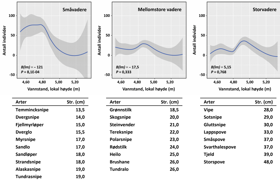
Figur 9: Sammenhengen mellom vannstand og småvader (venstre panel), mellomstore vader (midtre panel) og storvader (høyre panel). Modellen er basert på tellinger utført i perioden 15.7-15.9 for årene 1995-2001 og 2015-2018 ( n=88 ; feltdager) og beregnet ved hjelp av locally estimated scatterplot smoothing (loess). Den blå kurven viser modellen og det grå området 95%-konfidens-intervallet. B(lm) : lineært stigningstall med korresponderende P -verdi. Str.: minste oppgitte størrelse i centimeter i standardverk [12].
